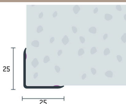
Ochranný rohový profil samolepiaci 25x25 mm, dĺžka 250 cm
