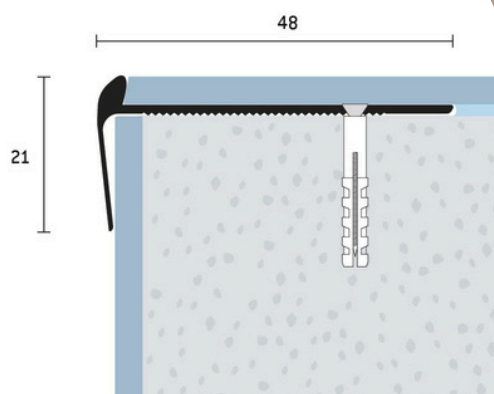
Schodová hrana vŕtaná 48x21 mm, hrúbka 5 mm, dĺžka 250 cm
